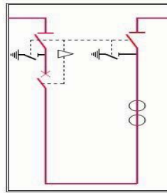
ŞEKİL - 7 BARA BAĞLAMA (KESİCİLİ KÜPLAJ) HÜCRETİ
