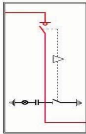
ŞEKİL - 5 YÜK AYIRICILI BARA BÖLME HÜC. (Yandan Çıkışı)
