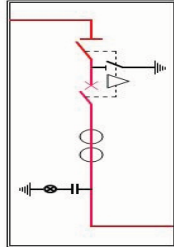
ŞEKİL - 9 KESİCİLİ BARA BÖLME HÜCRETİ (Yandan Çıkışı)
